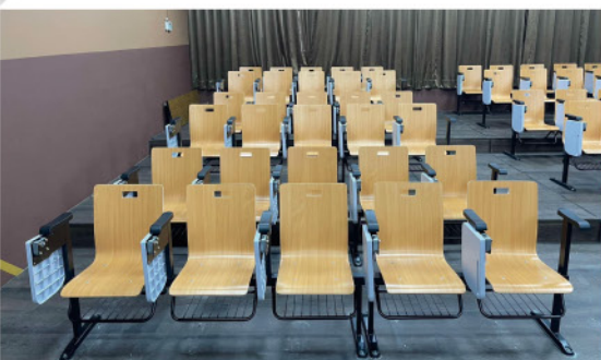
◆202I-1視聽連結椅 W580xD690xH860(mm)
