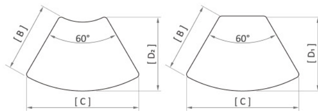
707a (內外圓弧)
