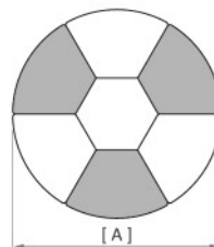
◆707Lb 扇形討論桌 (內直外圓) W900xD600xH750(mm)
