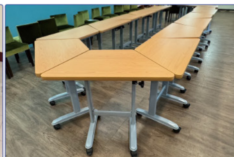
◆705Fm梯形桌(TPR輪) W1200xD600xH750(mm)
